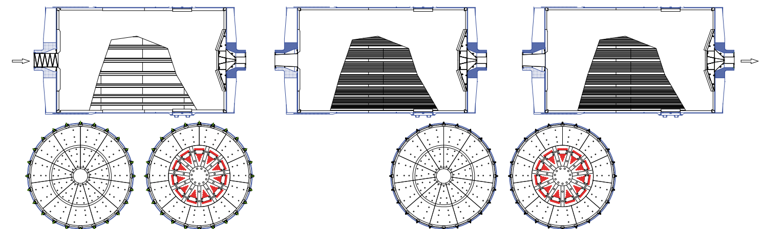
Testata di carico primo modulo 1st Module loading head Cabezal de carga primer modulo Tête de chargement premier module
