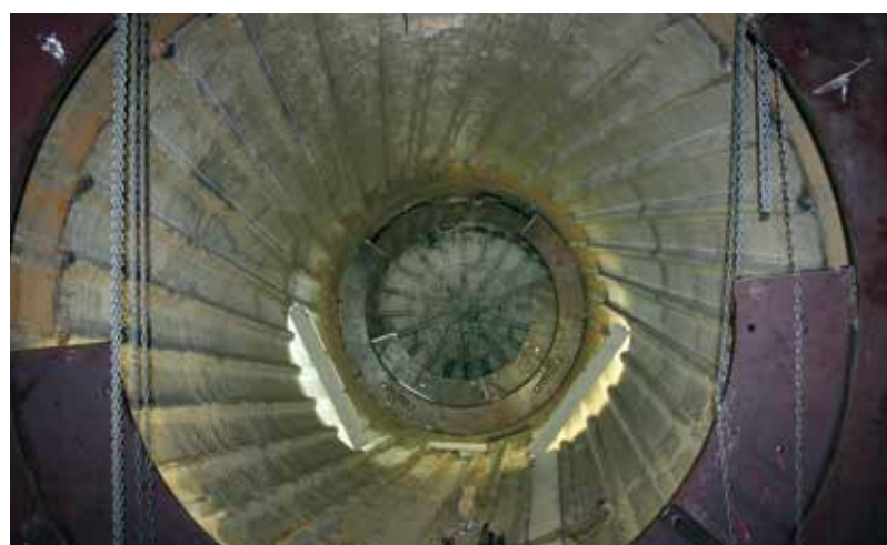
Assemblaggio di n. 2 anelli in acciaio all'interno del mulino.
