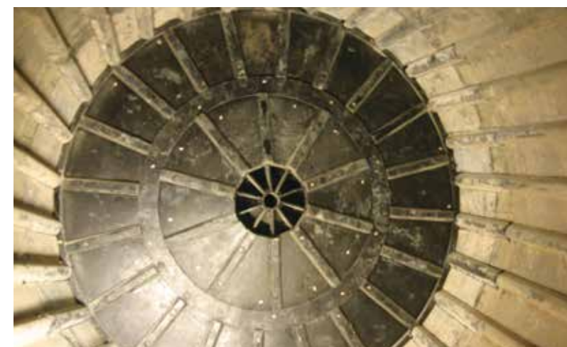
Montaggio della gomma sul diaframma e raccordo del rivestimento del cilindro contro al diaframma.
