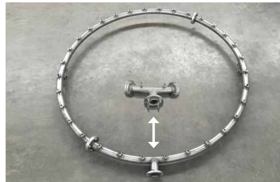
Corona di spruzzatura per atomizzatori con possibilità di averla con raccordo di ingresso intercambiabile e flangiata in due metà per facilitarne la pulizia. Spraying crown for spray driers with possibility of made it with interchangeable entry connection and flanged in two halves to ease its cleaning. Corona de pulverización para atomizadores con posibilidad de tenerla con conexión de entrada intercambiabile y con brida en dos mitades para facilitar su limpieza. Couronne de pulverisation pour atomiseurs avec possibilité de l'avoir avec connexion d'entrée interchangeable et avec bride en deux moitiés pour en faciliter le nettoyage.
