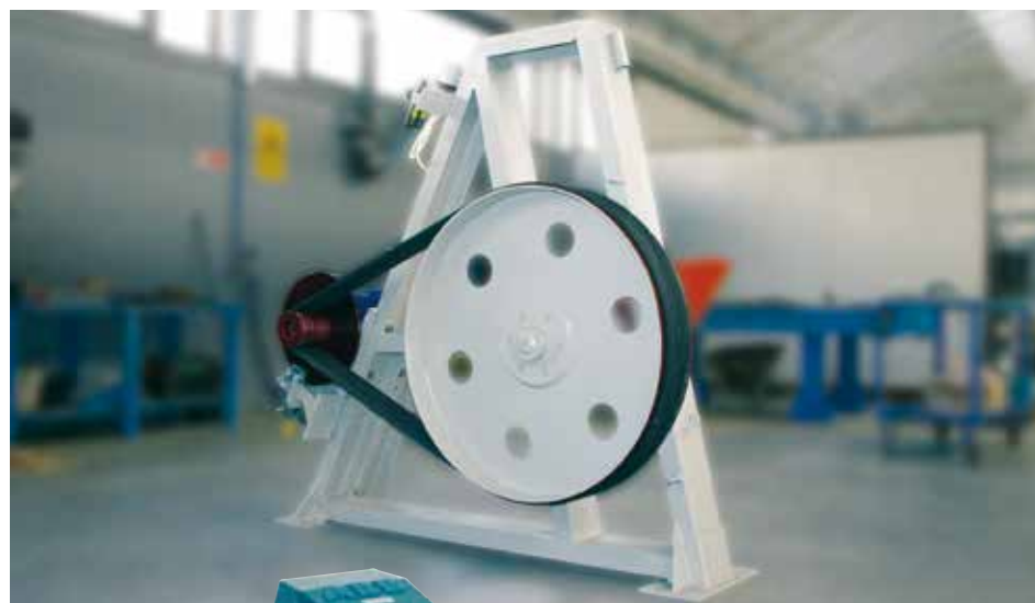
Dettaglio posteriore motorizzazione. Rear view of motorization unit. Detalle posterior motorización. Détail partie arrière motorisation.
