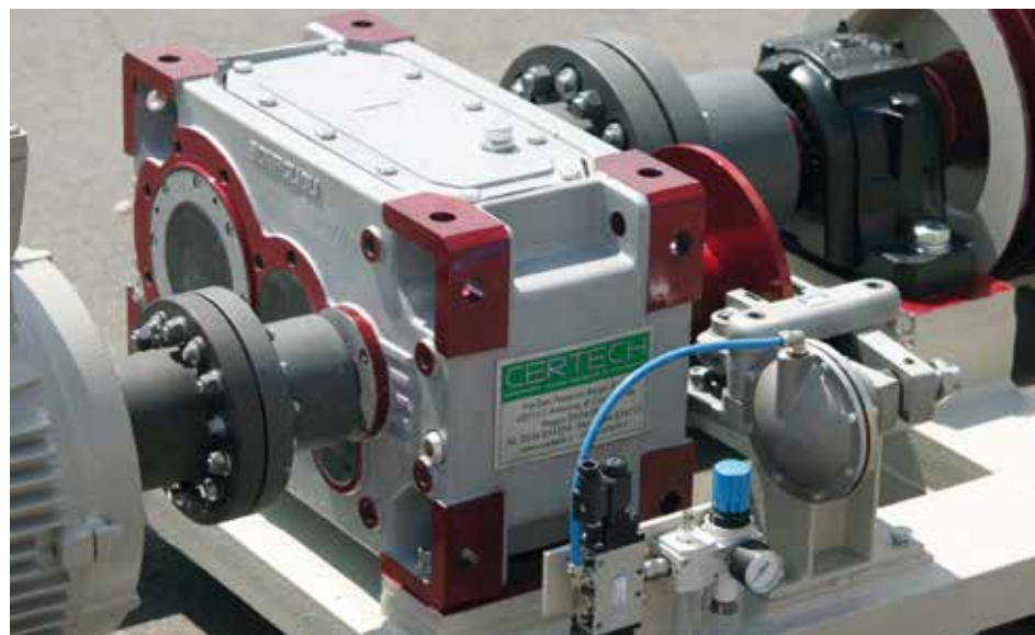
Motorizzazione tipo MRC 05. Dettaglio riduttore e gruppo frenante. MRC 05 motorization unit. Detail of reduction gear and braking group Motorizacion tipo MRC 05. Detalle reductor y grupo freno. Motorisation type MRC 05. Détail réducteur et groupe de freinage.
